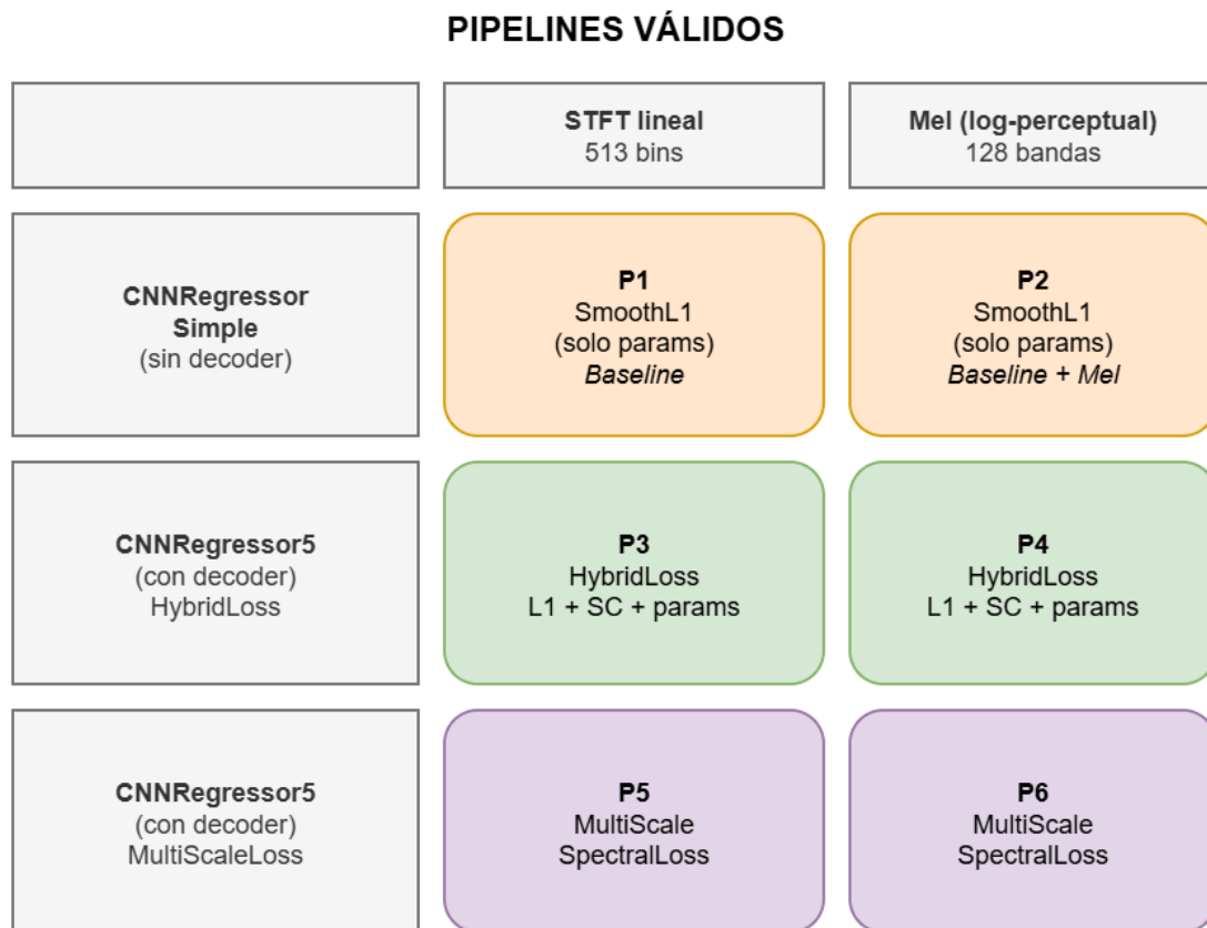
Figura 6.1: Representación de las diferentes combinaciones de Arquitecturas y Funciones de Pérdida.
